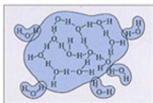
Normale molecola dell'acqua
